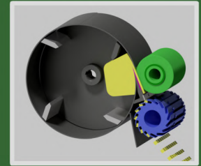
Schneiden von Würfeln mit Trennmesser, oberen Kreismessern und unteren Quermessern Cutting of cubes with block knife, upper circular knives and lower cross knives
