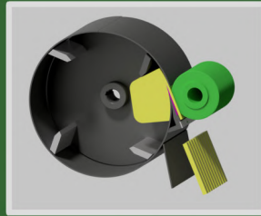
Schneiden von Streifen mit Trennmesser und oberen Kreismessern Cutting of strips with block knife and upper circular knives
